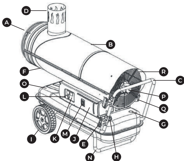
рис. 1. Устройство прибора
